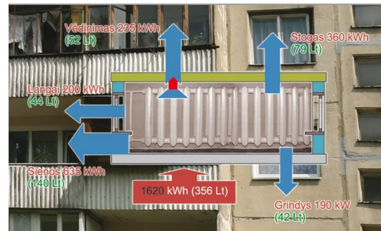
Nerenovuoto namo buto suvartoto šilumos kiekio šildymui, šilumos sklaidos ir mokėjimų struktūra
